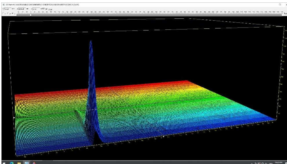
Slika 18. 3D kromatogram adalimumaba (koncentracija standardne otopine 500 µg/mL) nakon provedbe razgradnje na povišenoj temperaturi tijekom 48 sati.
