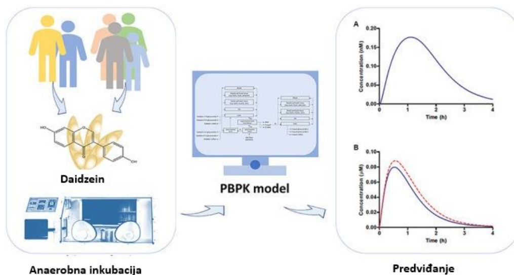
Slika 15. Fiziološki utemeljen farmakokinetički model za predviđanje mikrobne konverzije daidzeina u S-(-)ekvol, prilagođeno prema (9)
