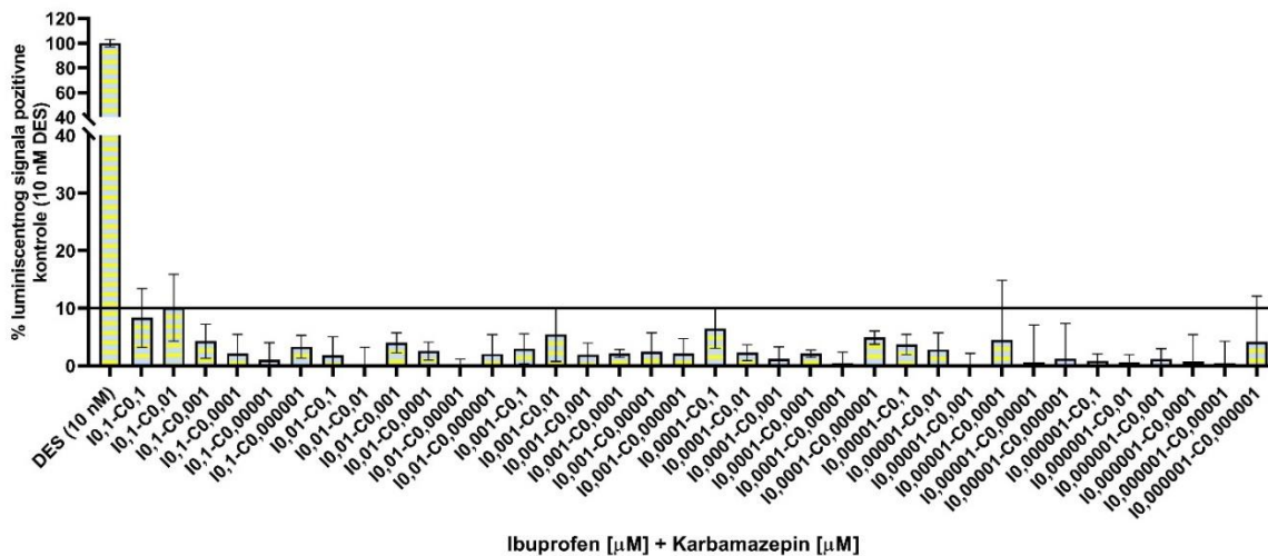
Slika 21. Aktivnost ER uzrokovana tretmanom smjesama ibuprofena i karbamazepina u koncentracijama od 1 \times 10^{-5} - 0,1 \mu\text{M} . Rezultati su prikazani kao % luminiscentnog signala pozitivne kontrole (10 nM) DES. Ukoliko je odaziv ispitivane kemikalije >10 % luminiscentnog signala pozitivne kontrole (označeno punom linijom na grafu), kemikalija se smatra endokrino disruptivnom s obzirom na djelovanje na ER. Prikazani rezultati dobiveni su iz triplikata dvaju ponovljenih eksperimenata.
