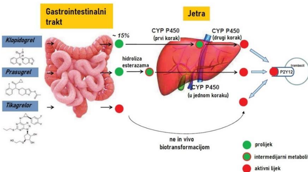
Slika 5. Mehanizam aktivacije P2Y 12 inhibitora
