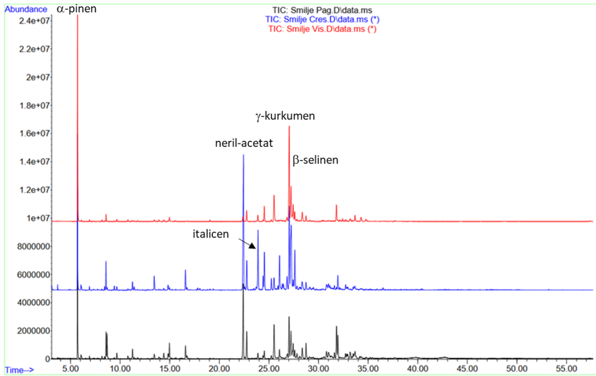
Slika 9. Usporedni prikaz kromatografskog profila eteričnih ulja sredozemnog smilja s otoka Visa, Cres i Paga
