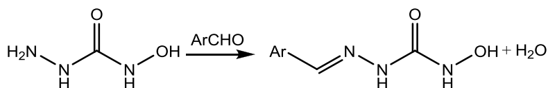
Shema 18. Schiffove baze 4-hidroksisemikarbazida
