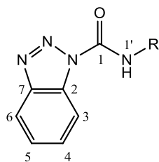
Tablica 9. ^{13}\text{C} NMR za 1-karbamoilbenzotriazole 7a-g
