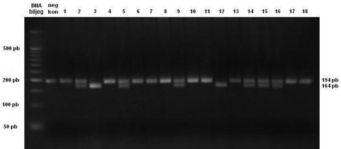
Slika 4.34. Elektroforeza produkata kidanja restriksijskim enzimom SmaI u 4 %-tnom agaroznom gelu. DNA biljeg = O'RangeRuler 50 bp DNA Ladder (Thermo Scientific); neg kon = negativna kontrola; linije 1, 4, 6, 7, 8, 10, 11, 13, 17 i 18 = AA genotip, linije 2, 5, 9, 14, 15 i 16 = AG genotip; linije 3 i 12 = GG genotip.
