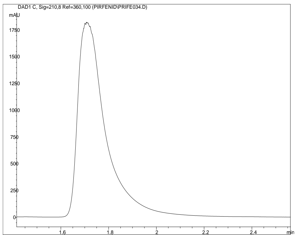
Slika 8. UV/ VIS kromatogram pirfenidona pri sastavu mobilne faze acetonitril: voda= 40:60.
