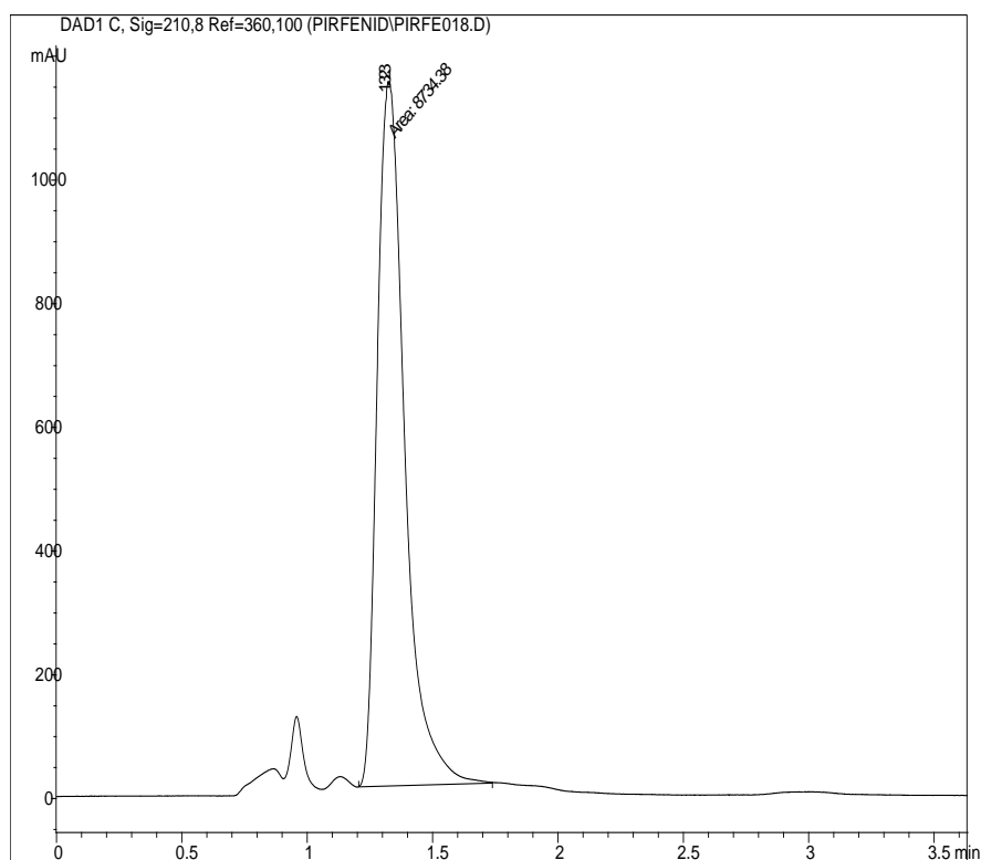
Slika 7. UV/ VIS kromatogram pirfenidona pri sastavu mobilne faze acetonitril:voda= 50:50.
