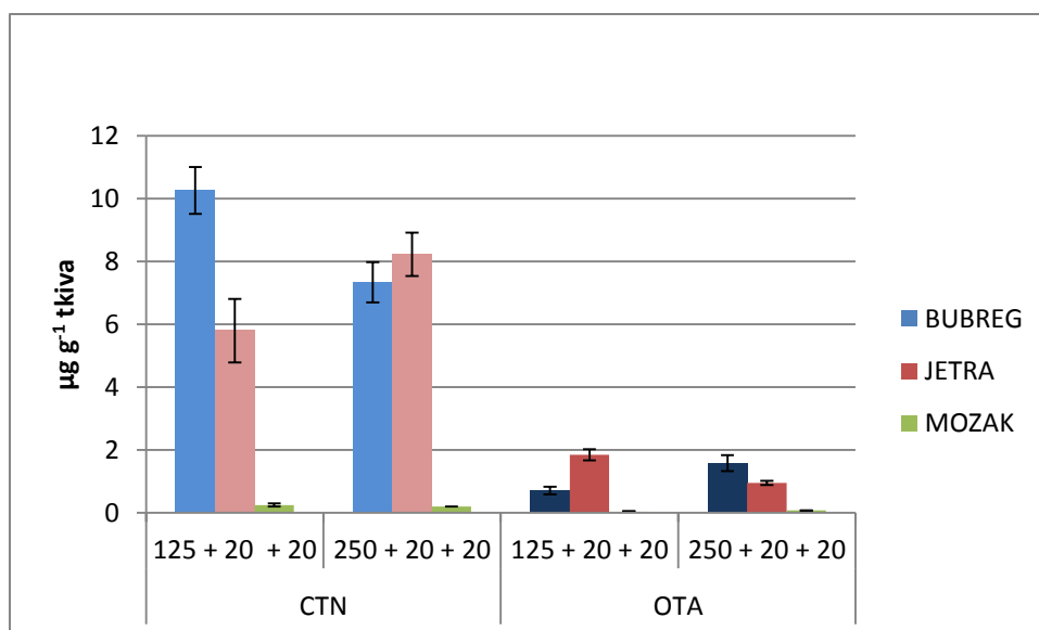
Slika 5-11 Koncentracije citrinina i okratoksina A u bubregu, jetri i mozgu kontrolnih životinja i životinja tretiranim s okratoksinom A (125 i 250 \mu\text{g kg}^{-1} tm) i resveratrolom (20 \text{mg kg}^{-1} ) tijekom 21 dan i citrininom (20 \text{mg kg}^{-1} ) tijekom posljednja dva dana pokusa. Rezultati su prikazani kao srednja vrijednost \pm standardna devijacija.
