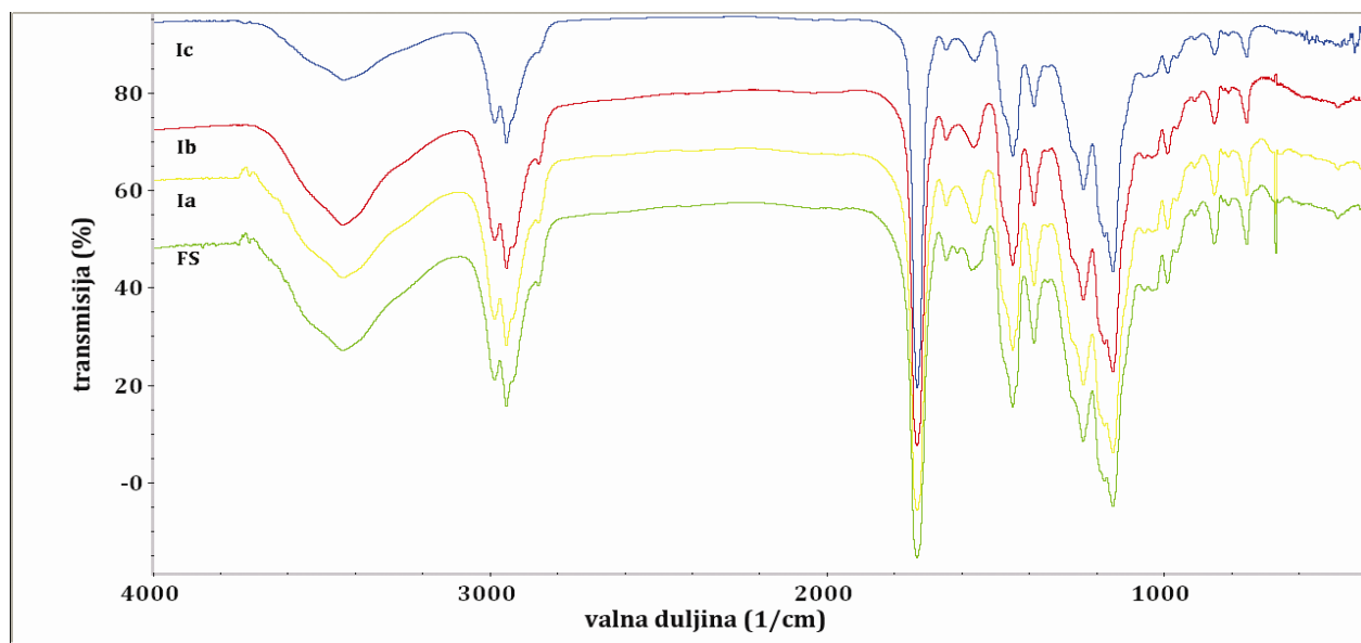
Slika 5 - 20. FTIR spektri mikročestica s omjerom lijeka i polimera 1 : 5 ( m/m ) sušenih raspršivanjem iz a) metanola; b) metanol-etanolske smjese (50 : 50, m/m ) i c) aceton-izopropanolske smjese (40 : 60, m/m ) u usporedbi s fizičkim smjesama (FS) lijeka i polimera
