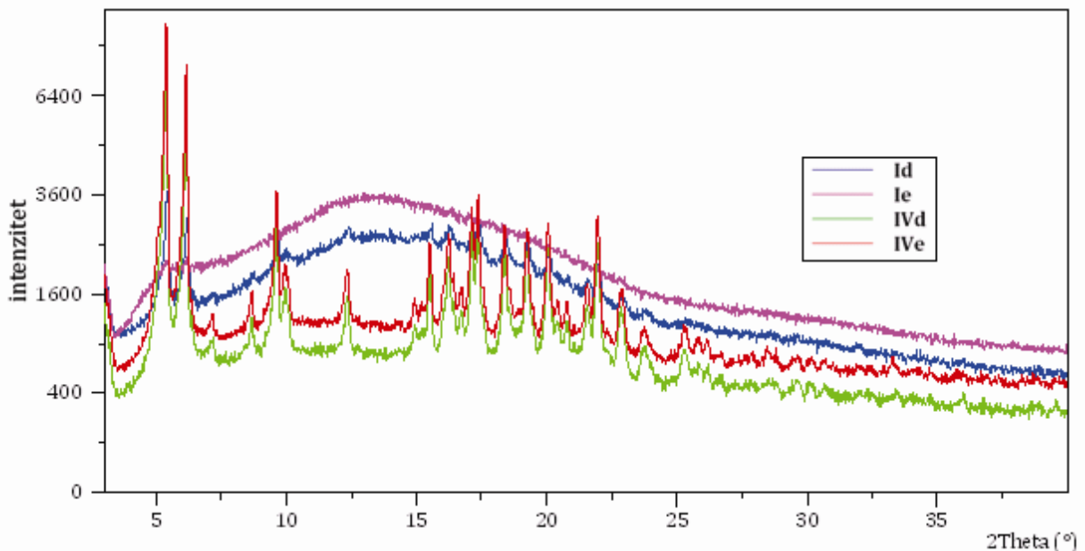
Slika 5 – 30. Difraktogram mikročestica s omjerom lijeka i polimera 2 : 1 i 5 : 1 ( m/m ) sušenih raspršivanje iz smjesa različitih fizičkih oblika lijeka i polimera
