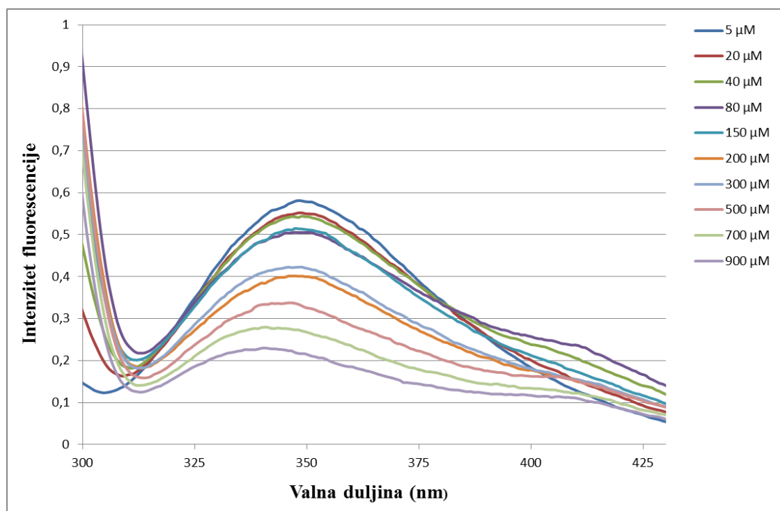
Slika 8.4.4. Fluorescencijski spektar albumina pri stalnoj koncentraciji (0.3 μM) i rasponu koncentracija CIT-AgNP od 5 do 900 μM u fosfatnom puferu.
