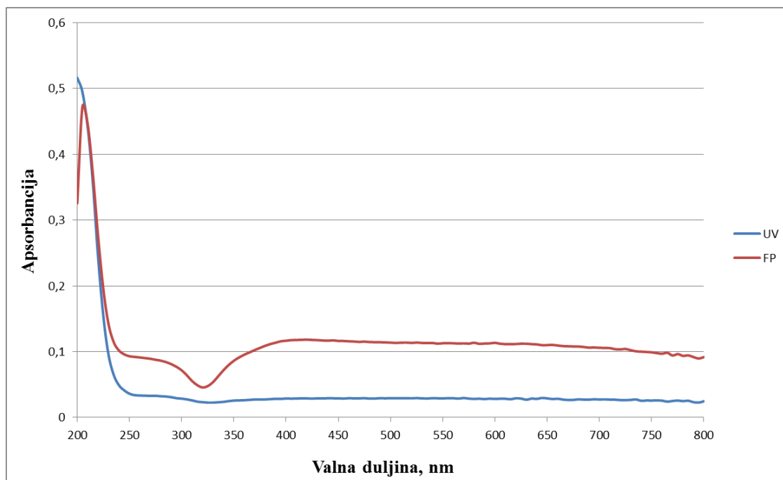
Slika 8.2.2. UV-Vis spektar CTA-AgNP (50 µM) u ultračistoj vodi (UV) i fosfatnom puferu (FP).
