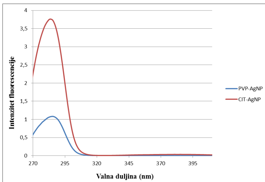
Slika 8.3.2. Fluorescencijski spektar PVP-AgNP i CIT-AgNP koncentracije 100 \mu\text{M} u ultračistoj vodi.
