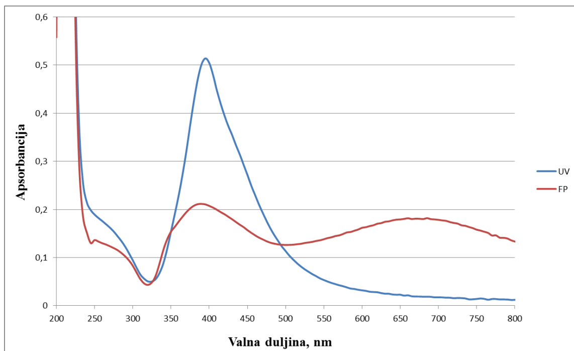
Slika 8.2.1. UV-Vis spektar PVP-AgNP (50 µM) u ultračistoj vodi (UV) i fosfatnom puferu (FP).
