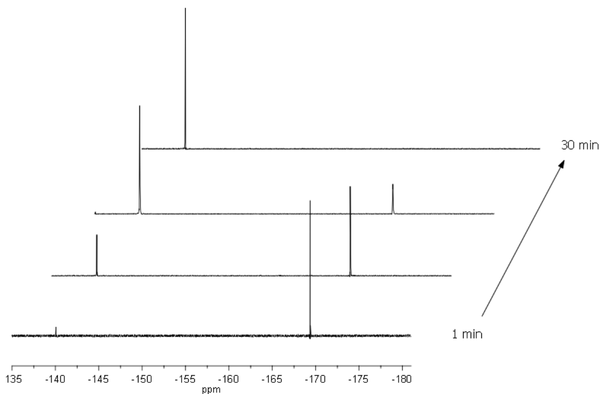
Slika 6. ^{19}\text{F} NMR spektroskopska analiza reakcije 5-FU i \text{HOCl} u vodi.
