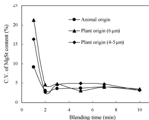
Slika 12. Utjecaj porijekla dobivanja magnezijeva stearata na ujednačenost njegove raspodjele u granulama. Na osi y prikazane se vrijednosti koeficijenta varijance dobivene iz 10 uzoraka.
