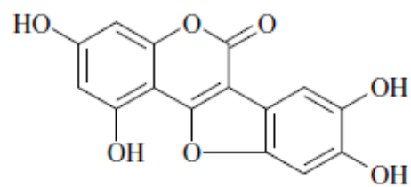
Desmetilvedelolakton
