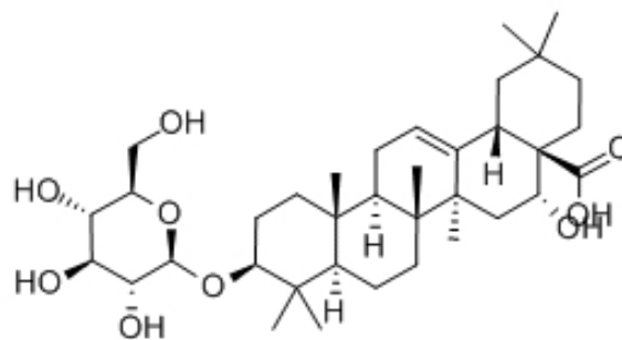
Ekliptasaponin A
