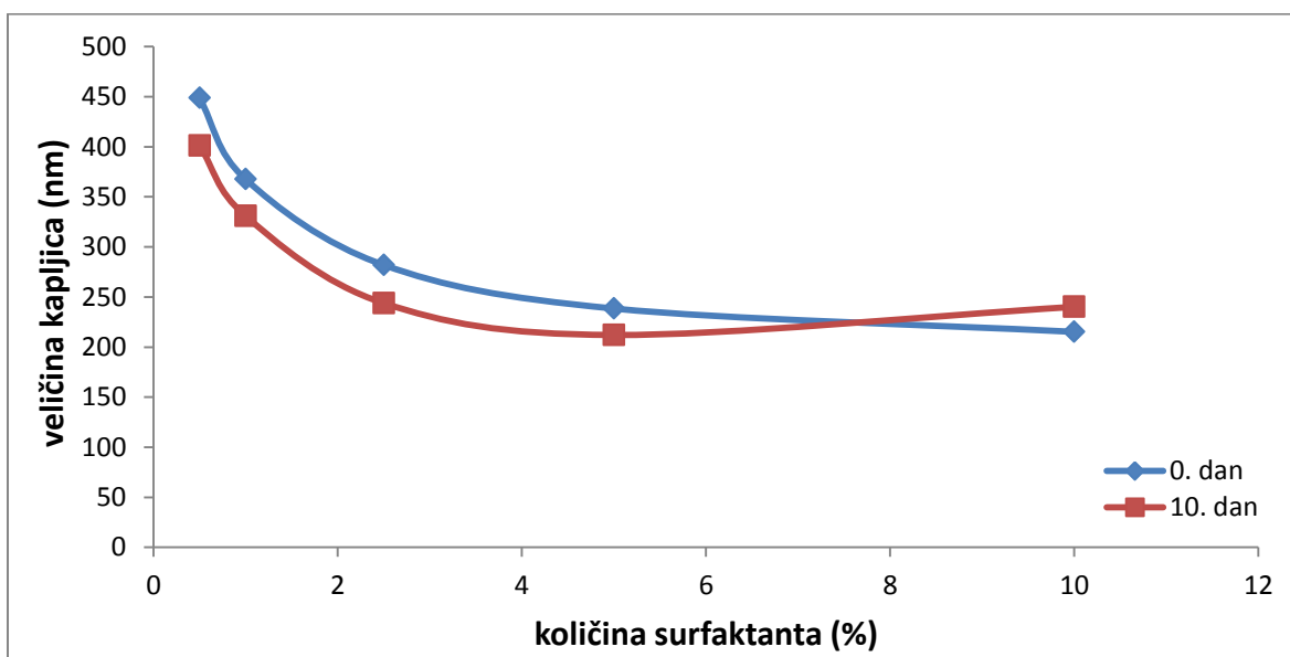
Slika 14. Ovisnost veličine kapljica ricinusova ulja o količini Polisorbata 80 u nanoemulziji.
