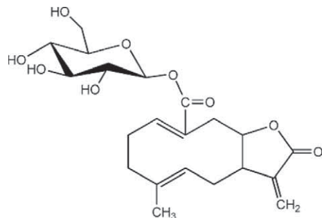
Slika 17. Struktura taraksinske kiseline s \beta -D-glukozom (79)
