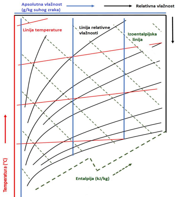
Slika 2. Molliereov dijagram – crvene linije predstavljaju izoterme, zelene isprekidane linije su izoentalskijske linije. Apsolutna vlažnost zraka prikazana je plavim vertikalnim linijama, dok je relativna vlažnost zraka prikazana crnim zakrivljenim linijama. Tlak vlažnog zraka utječe na karakteristike dijagrama, pa je svaki Molliereov dijagram napravljen tako da prikazuje uvjete pri jednoj specifičnoj vrijednosti tlaka zraka.
