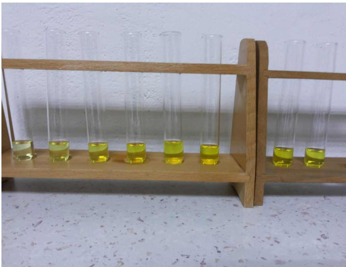
Slika 9. Pripremljena razrjeđenja kvercetina tijekom inkubacije s \text{AlCl}_3
