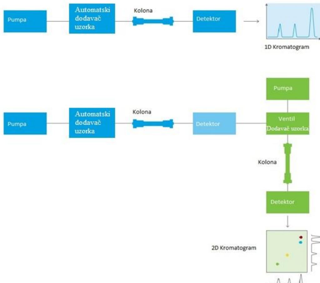
Slika 4: Usporedba jednodimenzionalne i dvodimenzionalne kromatografije (Carr i Stoll, 2015)
