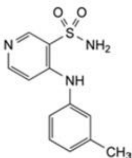
B. 4-[(3-metilfenil)amino]piridin-3-sulfonamid
