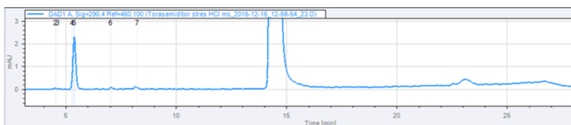
Slika 24: Kromatogram nakon izlaska iz prve dimenzije uzorka torasemida razgrađivanog u kiselim uvjetima, s označenim alikvotima skupljenima za drugu dimenziju
