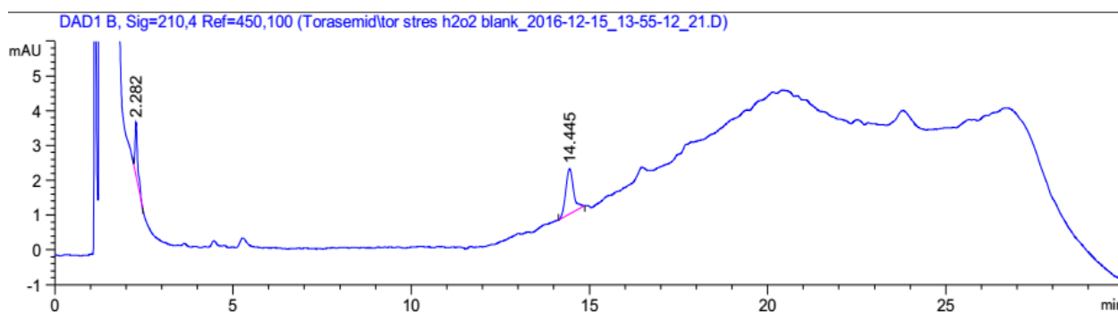
Slika 18: Kromatogram slijepog uzorka bez torasemida s H 2 O 2
