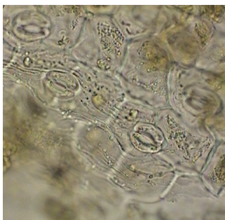
Slika 14. Dijacitične puči
