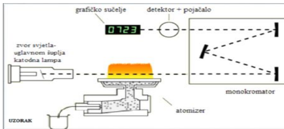
Slika 5. Princip FAAS (izvor: Amidžić Klarić, 2016)
