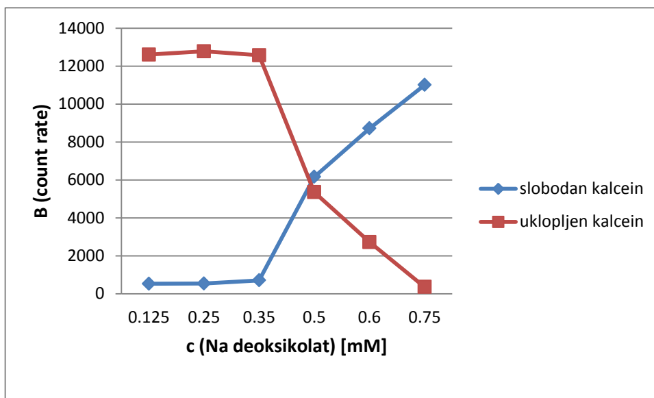
Slika 22. Ovisnost preeksponecijalnih faktora (B) o koncentraciji natrijevog deoksikolata nakon 180 minuta inkubacije
