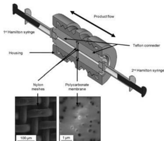
Slika 5. Shematski prikaz ručnog mini-ekstrudera ( http://www.jpharmsci.org )
