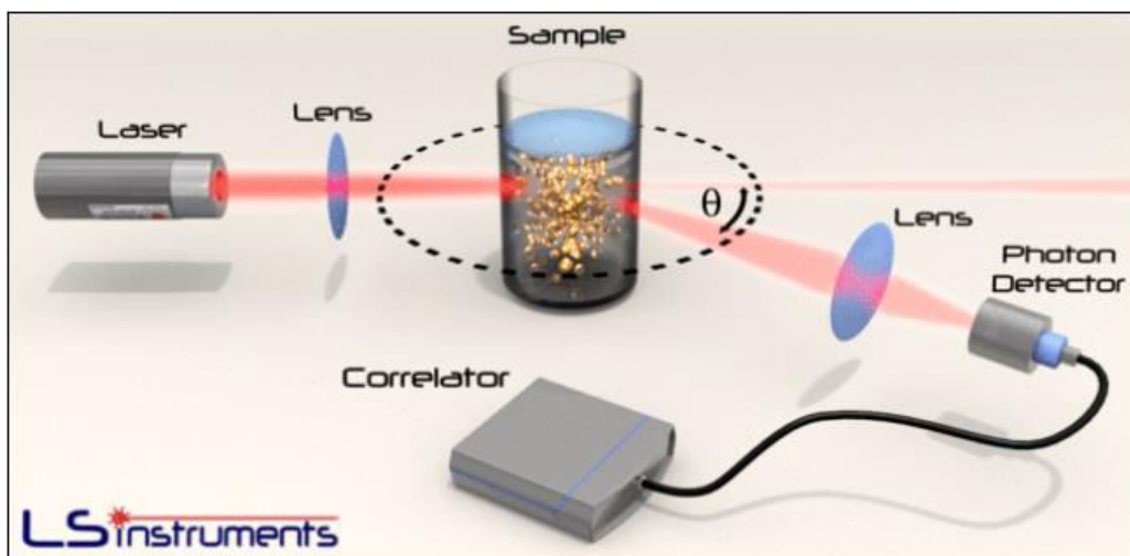
Slika 6. Shematski prikaz rada PCS uređaja ( http://www.lsinstruments.ch )
