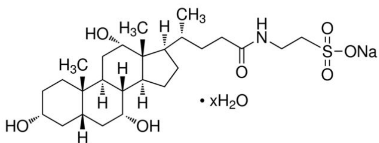
Slika 12. Na-taurokolat hidrat ( www.sigmaldrich.com )
