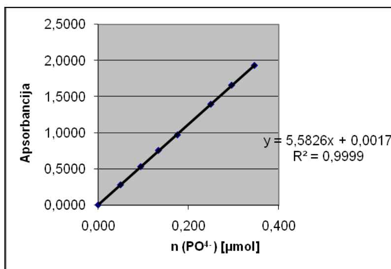
Slika14. Kalibracijski pravac otopine fosfatnog pufera
