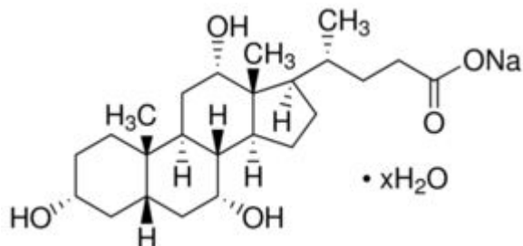
Slika 10. Na-kolat hidrat ( www.sigmaldrich.com )
