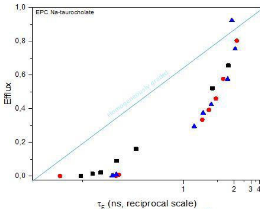
Slika 30. Ovisnost količine oslobođenog kalceina ( E , efflux ) o vremenu života uklopljenog kalceina ( \tau_E )
