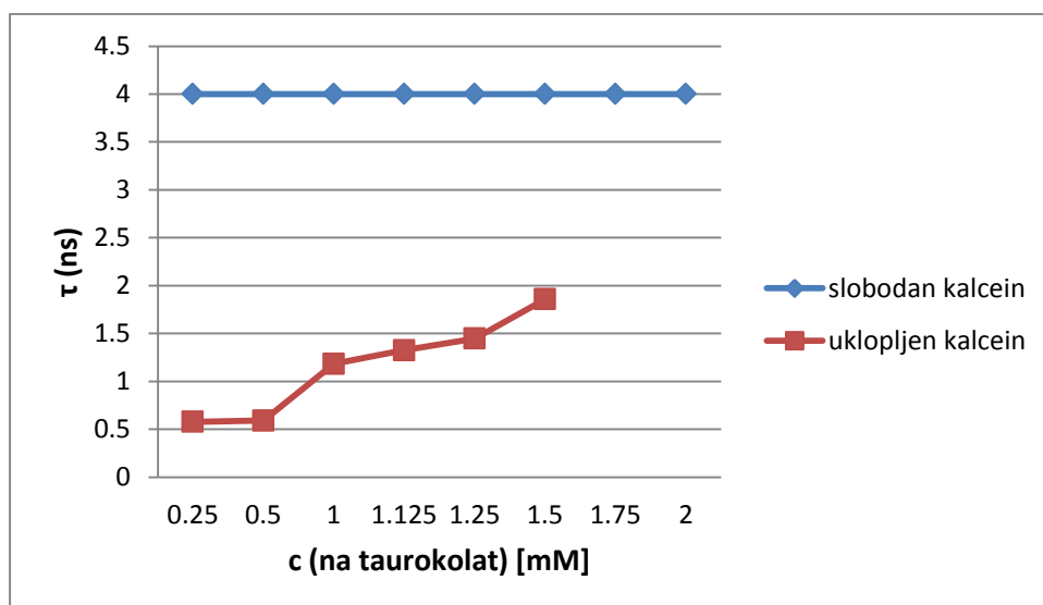
Slika 28. Ovisnost vremena života fluorescencije ( \tau ) o koncentraciji Na taurokolata nakon 180 min inkubacije
