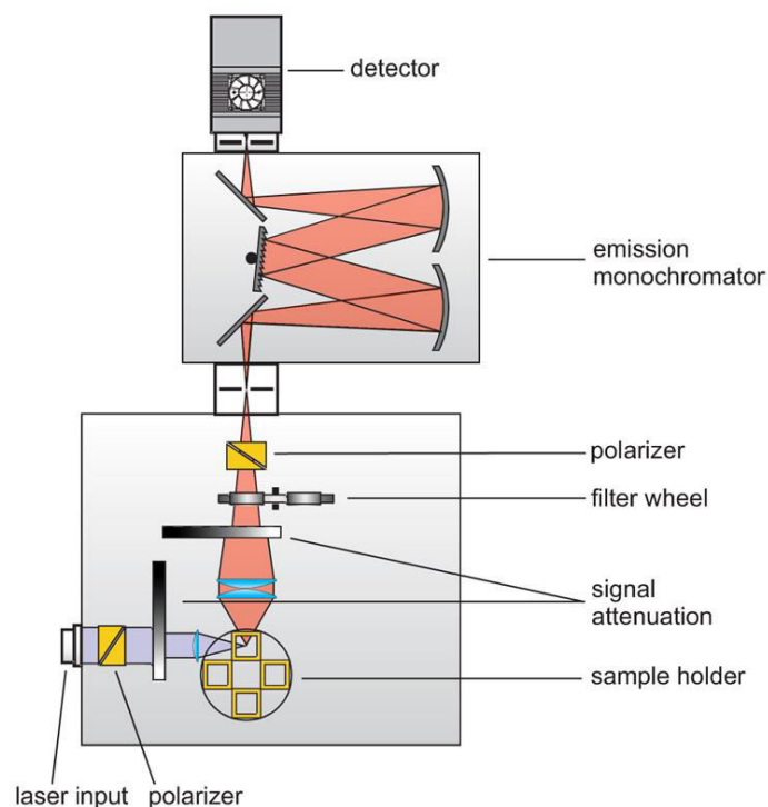
Slika 9. Shemtski prikaz uređaja za mjerenje vremena života fluorescencije ( www.picoquant.com )
