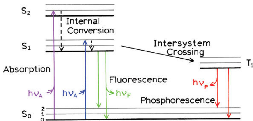
Slika 7. Energetski dijagram koji opisuje fluorescenciju i fosforescenciju (Jablonski dijagram) (Lakowicz, 2010)
