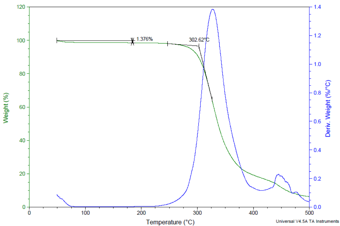
Slika 9. Termogram mikročestica PVA 8-88 pripravljenih sušenjem raspršivanjem
