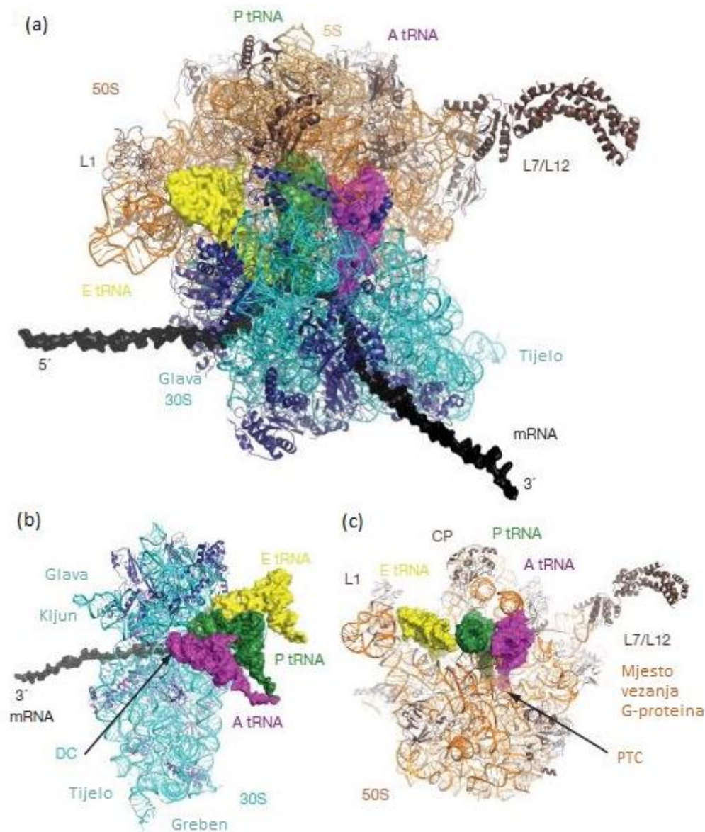
Slika 1.1.1.1.1. Struktura ribosoma. (a) Prikaz ribosoma 70S s mRNA i tRNA u mjestima A, P i E. (b) podjedinice 30S, (c) i podjedinice 50S. Podjedinica 30S prikazana je plavom, a podjedinica 50S narančastom bojom, pri čemu su proteinski dijelovi prikazani tamnije, a rRNA svjetlije. mRNA je prikazana sivom bojom, dok su tRNA s obzirom na mjesto koje zauzimaju prikazane ljubičastom (A-mjesto), zelenom (P-mjesto) i žutom (E-mjesto) bojom (preuzeto i prilagođeno iz Schmeing i Ramakrishnan, 2009).
