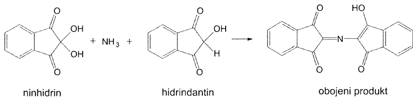
Slika 7. Ninhidrijska reakcija (23)
