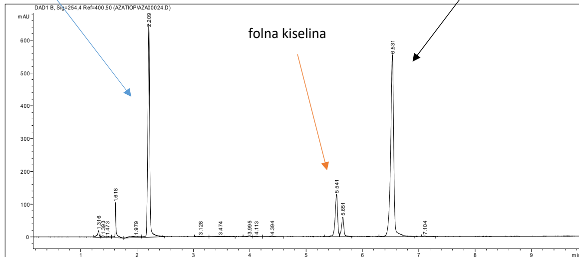
Slika 3. Kromatogram uzorka "umjetne plazme" u koju su dodane standardne otopine standarda: azatioprin, folna kiselina i 6-tiogvanin (6-TG).
