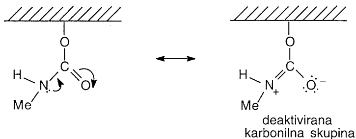
Slika 6. Stabilizacija intermedijera karbamoila i enzima
