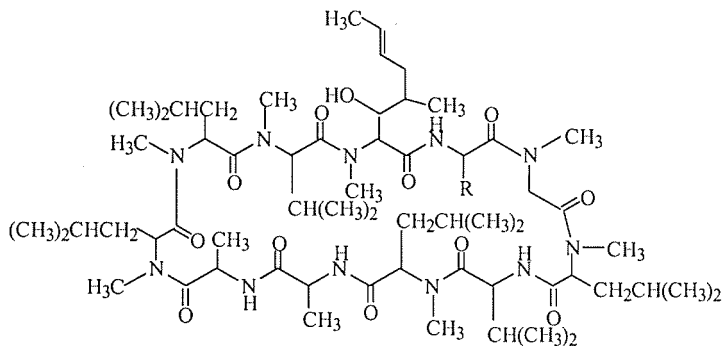
Slika 2. Ciklosporin A
