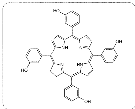
Slika 6. Temoporfin.
