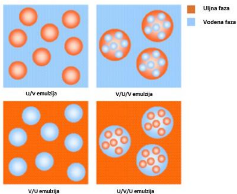
Slika 4. Tipovi emulzija (36)
