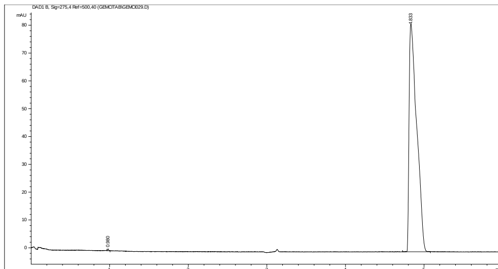
Slika 14. Elektroferogram smjese standardnih otopina gemcitabina (100 µg/ml) i njegovog onečišćenja citozina (190 µg/ml), na valnoj duljini 275 nm.
