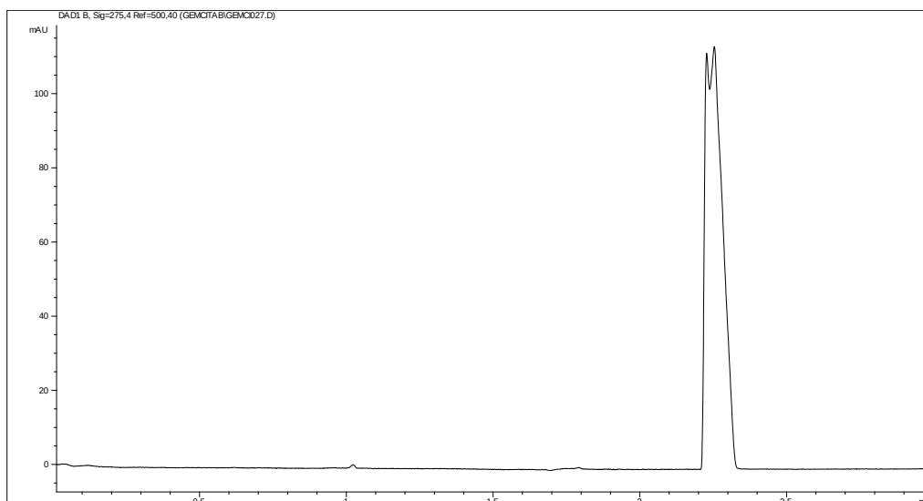
Slika 15. Elektroferogram smjese standardnih otopina gemcitabina (100 µg/ml) i njegovog onečišćenja citozina (190 µg/ml), na valnoj duljini 275 nm.
