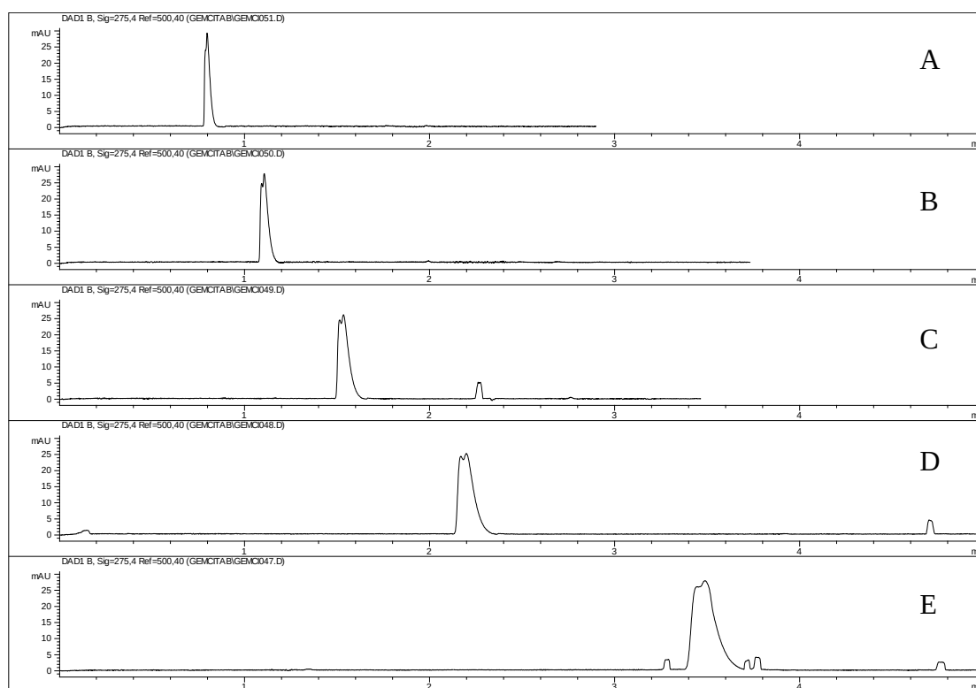
Slika 18. Elektroferogrami smjese standardnih otopina gemcitabina (50 µg/ml) i njegovog onečišćenja citozina (50 µg/ml), na valnoj duljini 275 nm, uz promjenu napona: (A) 30 kV, (B) 25 kV, (C) 20 kV, (D) 15 kV, (E) 10 kV.
