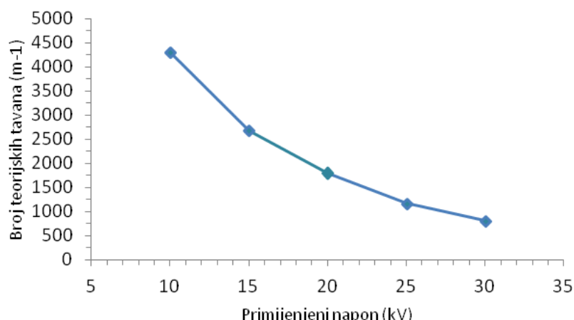
Slika 21. Utjecaj primijenjenog napona na učinkovitost metode za gemcitabin (50 µg/ml).
