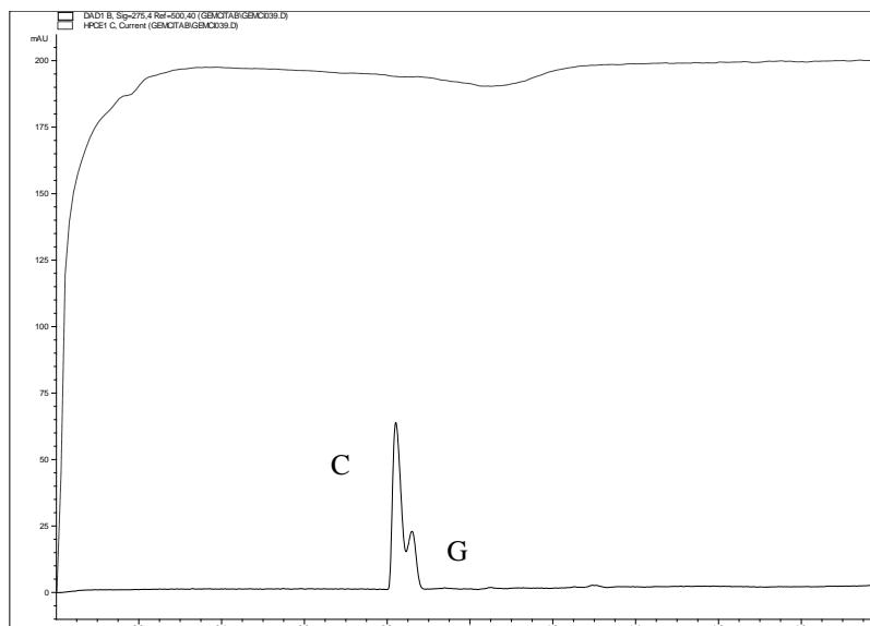
Slika 17. Elektroferogram smjese standardnih otopina gemcitabina (70 \mu\text{g/ml} ) i njegovog onečišćenja citozina (90 \mu\text{g/ml} ), na valnoj duljini 275 nm te prikaz povišenja jakosti struje (200 \mu\text{A} ).
