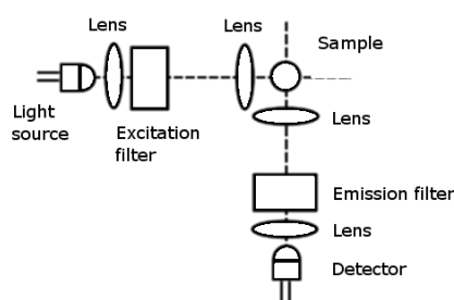
Slika 6. Shema fluorimetra
