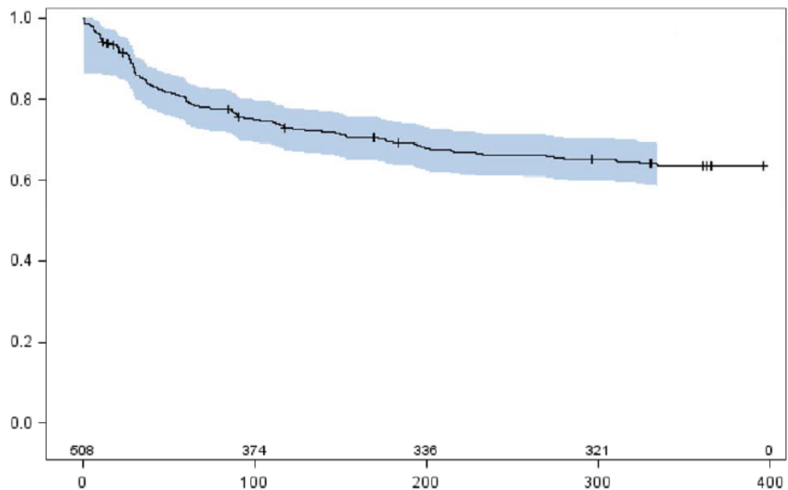
Slika 1: Kaplan-Meierova krivulja s 95% Hall-Wellner trakama za cijelu ispitivanu populaciju. Na x-osi se nalaze dani i populacija u riziku za promjenu dok je na y-osi postotak populacije koji nije imao promjenu.
