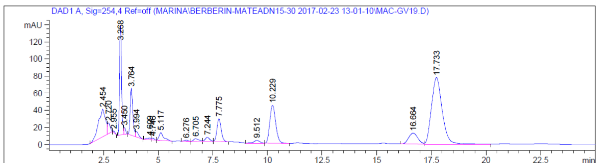
Slika 8. Kromatogram uzorka MAC-GV19 na 254 nm
