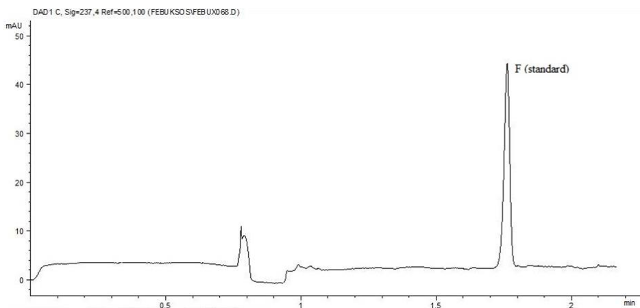
Slika 10. Elektroferogram standardne otopine febeksostata (F (standard), 50 µg/mL).
